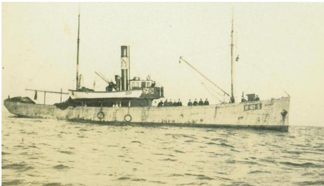
Bilde viser SS Sunde. Bygget i 1869. Lengde 105,1 fot, bredde 19,0 fotdybde 10,7 fot. Damp 190 hk. Eier Chr Bjelland & Co, Stavanger.
